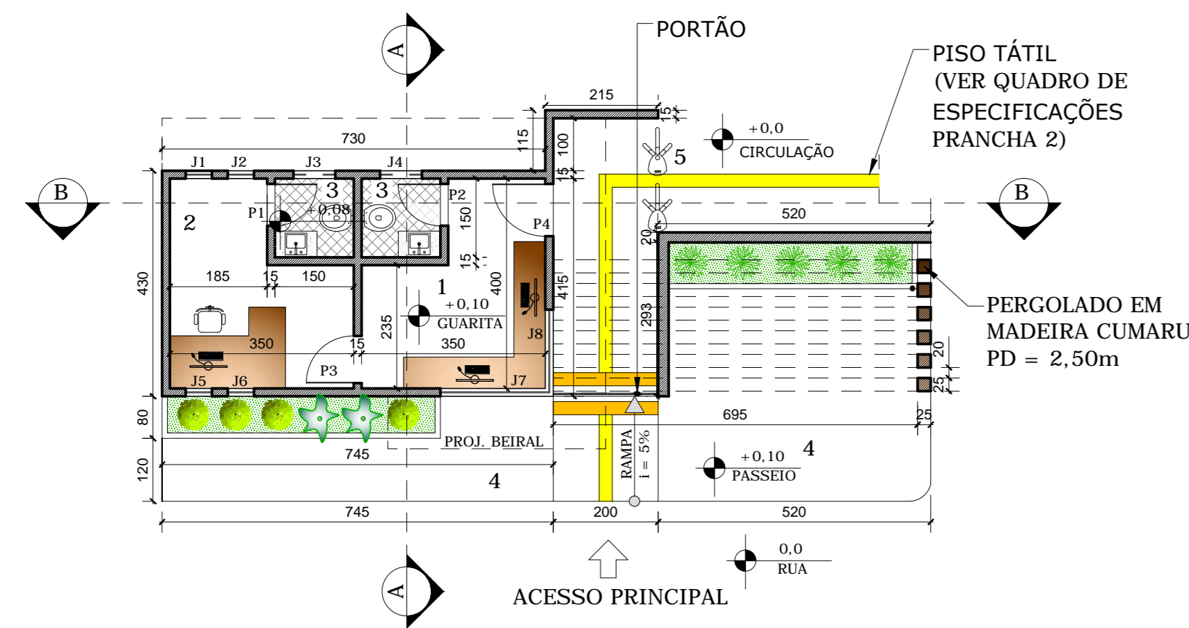
PLANTA BAIXA GUARITA ESCALA 1:100
