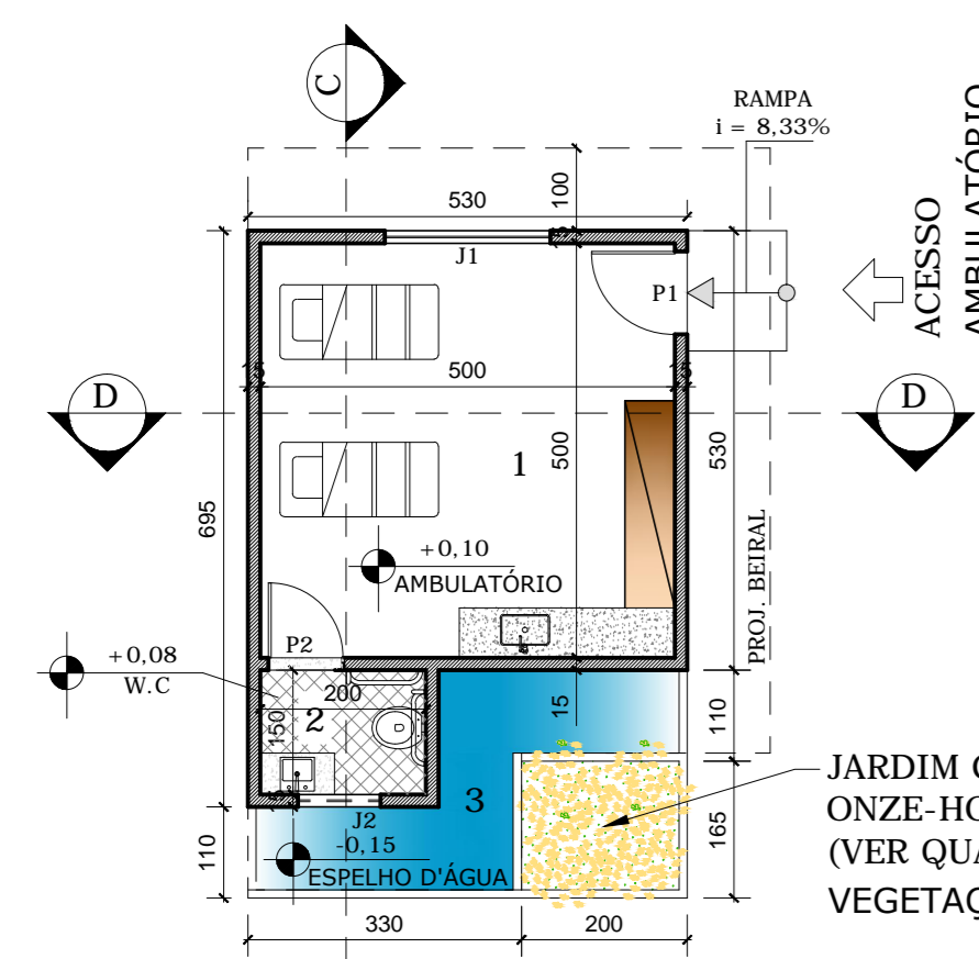
PLANTA BAIXA AMBULATÓRIO ESCALA 1:100
