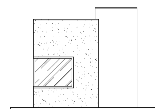
FACHADA GUARITA-F2 ESC.....1/100
