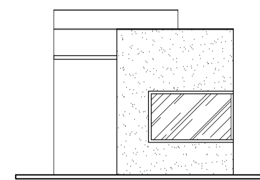
FACHADA GUARITA-F1 ESC.....1/100
