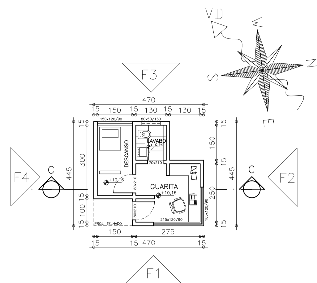
PLANTA BAIXA GUARITA 01-02 ESC.....1/100
