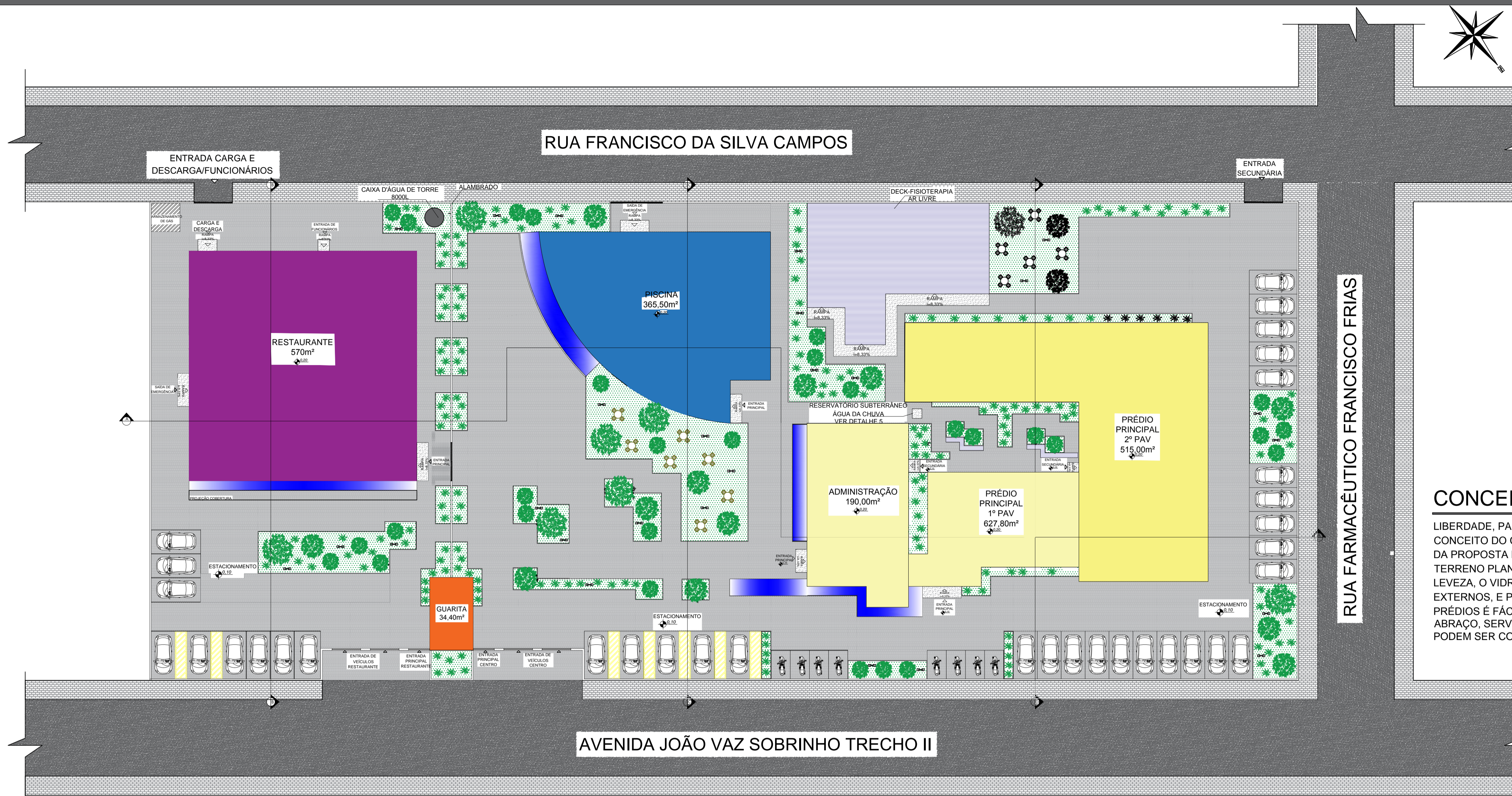
PLANTA DE IMPLANTAÇÃO/SITUAÇÃO ESCALA 1:250
