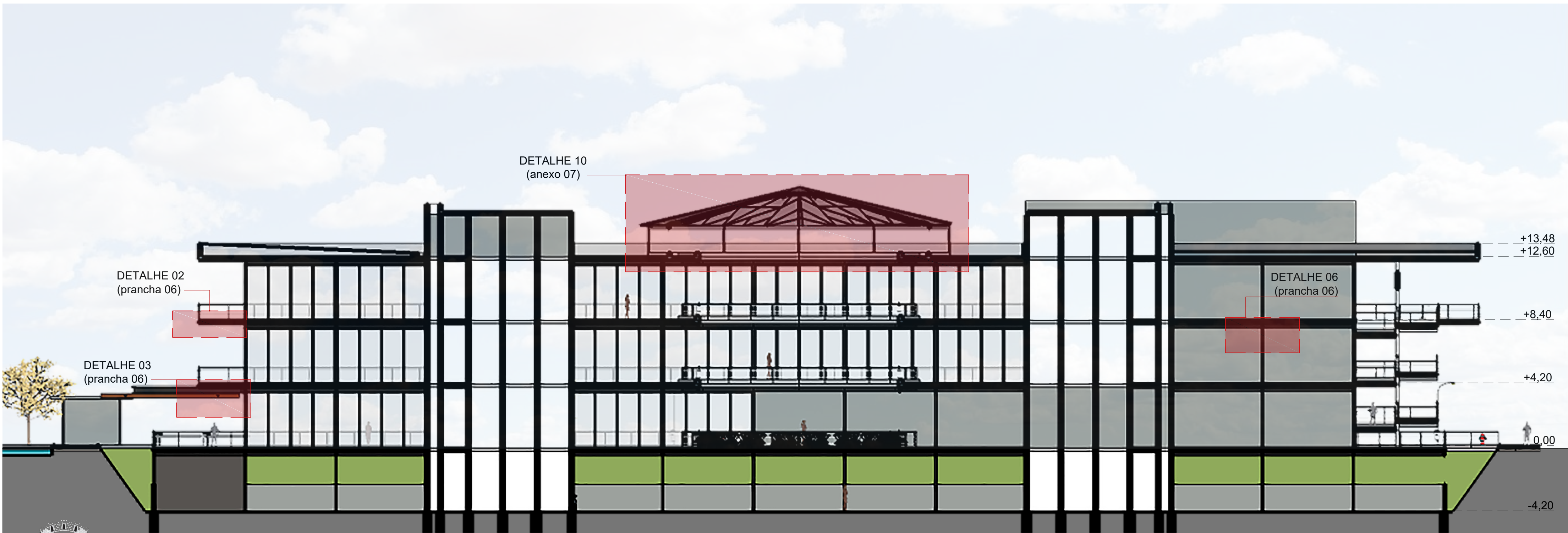
CORTE LONGITUDINAL AA | ESCALA 1:175
