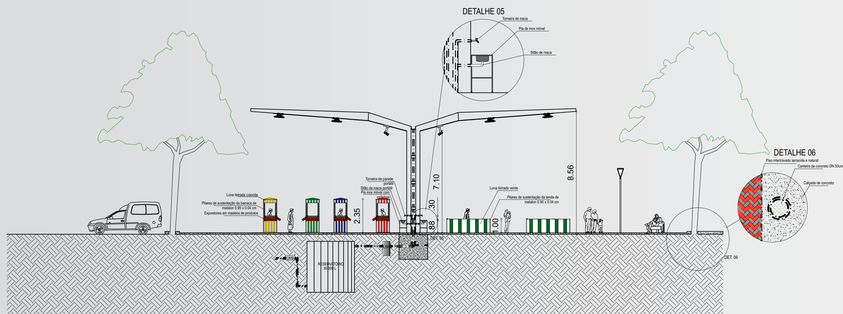
CORTE - COBERTURA ESC 1/150
