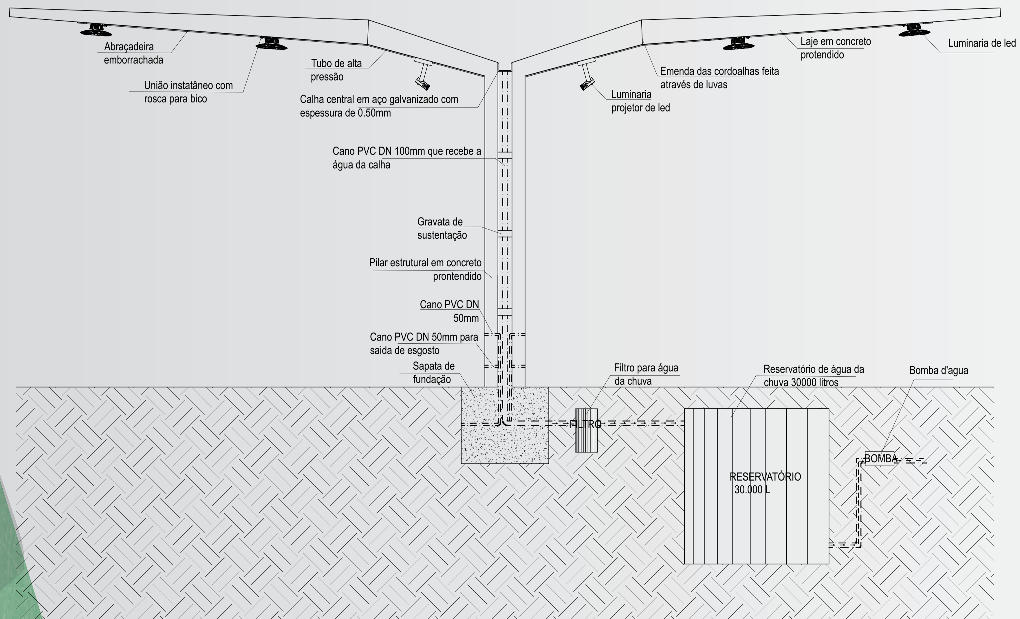
DETALHE - COBERTURA ESC 1/50
