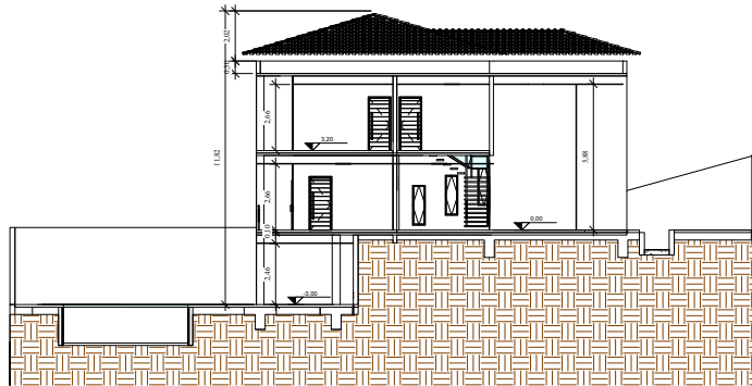
3 Corte 3 ESCALA - 1 : 100
