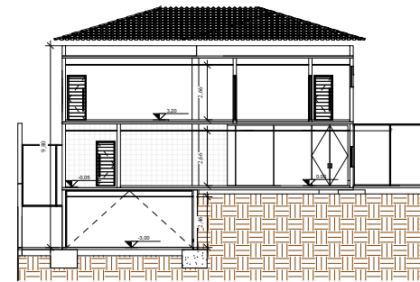
1/100 6 Corte 2 ESCALA - 1 : 100
