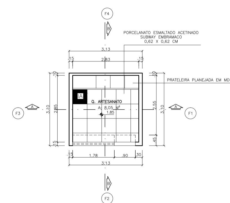
PAGINAÇÃO - QUIOSQUE ARTESANATO MODELO PADRÃO ESC: 1/75 M: ÍNDICE DE ASSENTAMENTO DO REVESTIMENTO C.N.R: 0,00 F: FACHADA OBS.: VER TABELAS - PÁGINA 06
