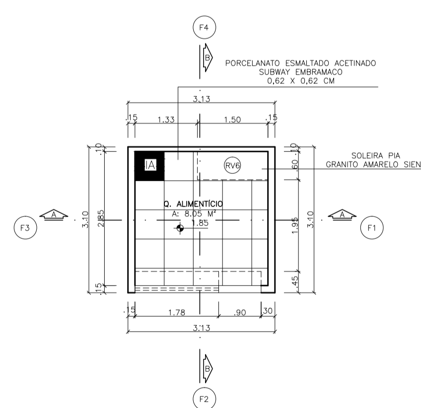
PAGINAÇÃO - QUIOSQUE ALIMENTÍCIO MODELO PADRÃO ESC: 1/75 M: ÍNDICE DE ASSENTAMENTO DO REVESTIMENTO C.N.R: 0,00 F: FACHADA OBS.: VER TABELAS - PÁGINA 06
