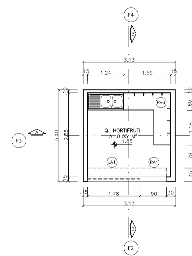
PLANTA - QUIOSQUE HORTIFRUTI MODELO PADRÃO ESC: 1/75 C.N.R: 0,00 F: FACHADA OBS.: VER TABELAS - PÁGINA 06
