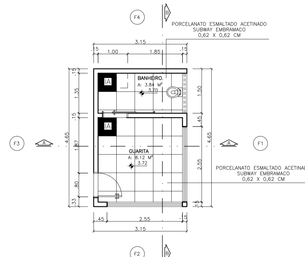
PAGINAÇÃO - GUARITA E MONITORAMENTO ESC: 1/75 M: ÍNDICE DE ASSENTAMENTO DO REVESTIMENTO C.N.R: 0,00 F: FACHADA OBS.: VER TABELAS - PÁGINA 06
