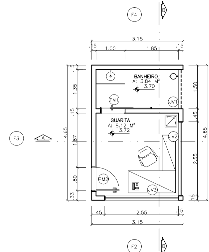
PLANTA - GUARITA E MONITORAMENTO ESC: 1/75 C.N.R: 0,00 F: FACHADA OBS.: VER TABELAS - PÁGINA 06
