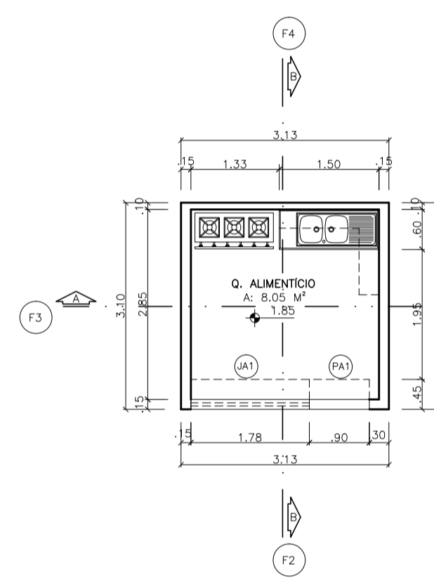
PLANTA - QUIOSQUE ALIMENTÍCIO MODELO PADRÃO ESC: 1/75 C.N.R: 0,00 F: FACHADA OBS.: VER TABELAS - PÁGINA 06
