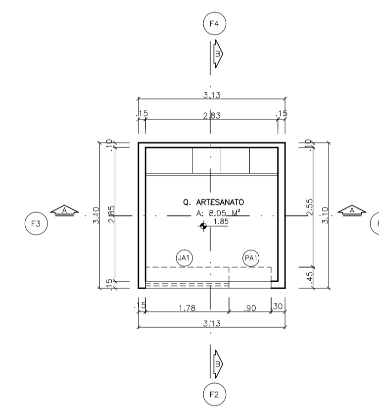
PLANTA - QUIOSQUE ARTESANATO MODELO PADRÃO ESC: 1/75 C.N.R: 0,00 F: FACHADA OBS.: VER TABELAS - PÁGINA 06
