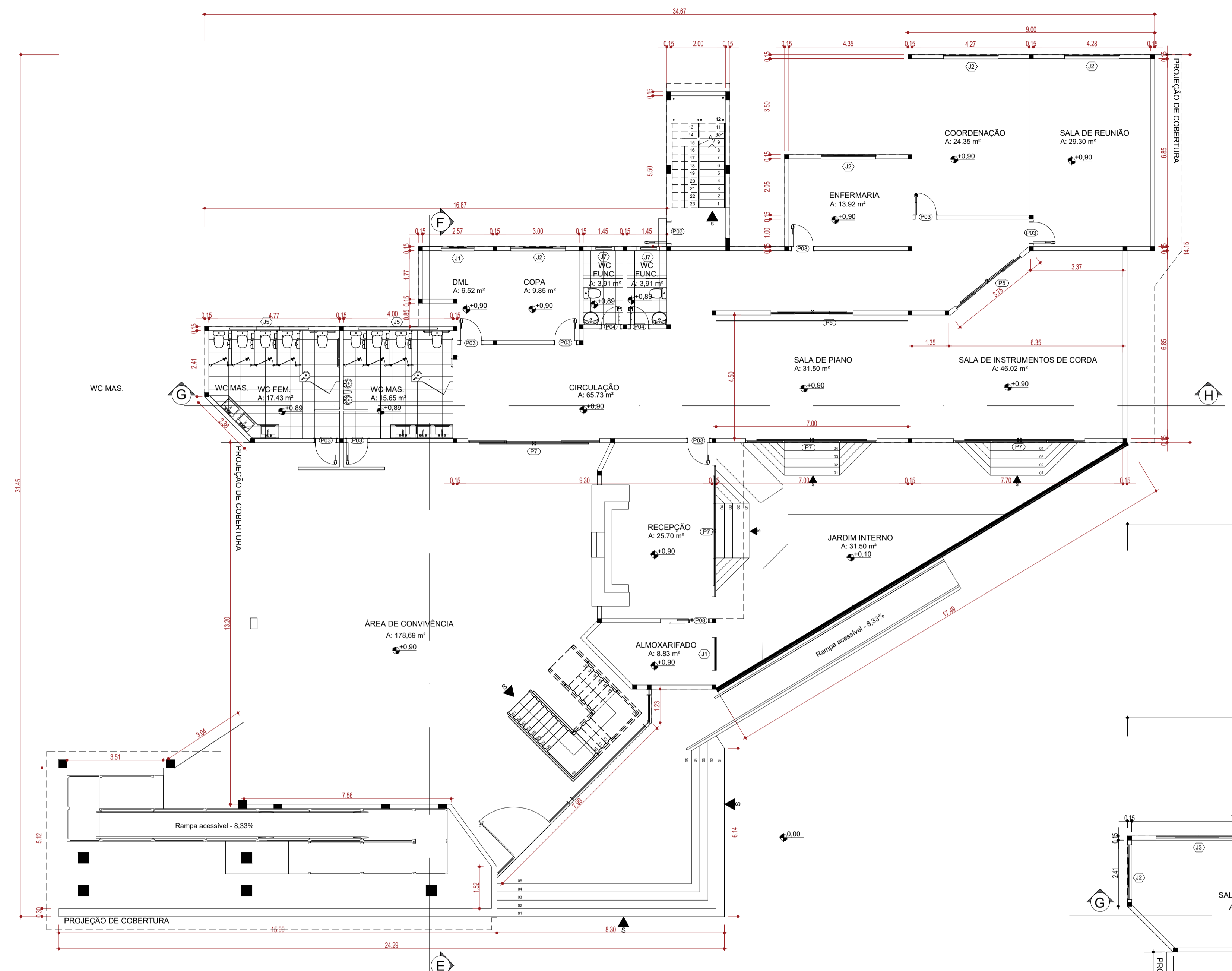
PLANTA BAIXA TÉRREO ESCOLA DE MÚSICA ESCALA 1:100
