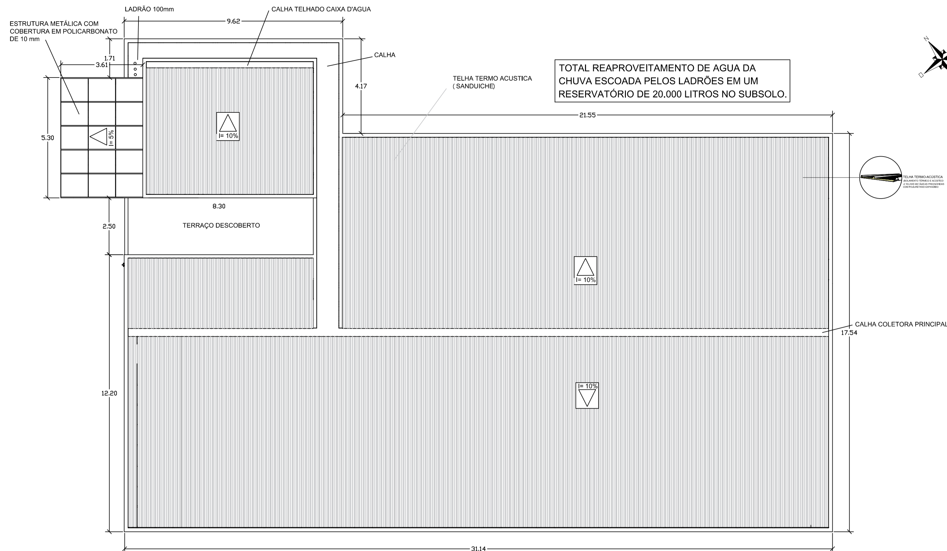
PLANTA DE COBERTURA AUDITÓRIO ESCALA 1:100
